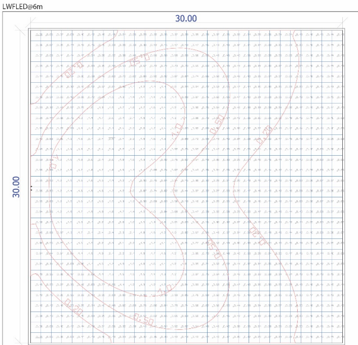
Scale: 1 : 200
